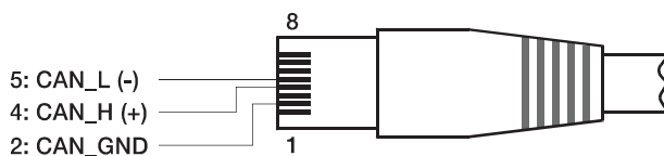
Rysunek 6.5: Schemat złącza CAN
