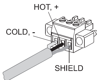
Rysunek 6.2: Kable symetryczne
