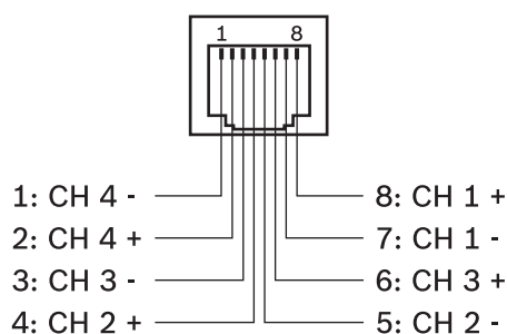
Rysunek 6.1: Przyporządkowanie styków gniazda LINE IN 1-4
